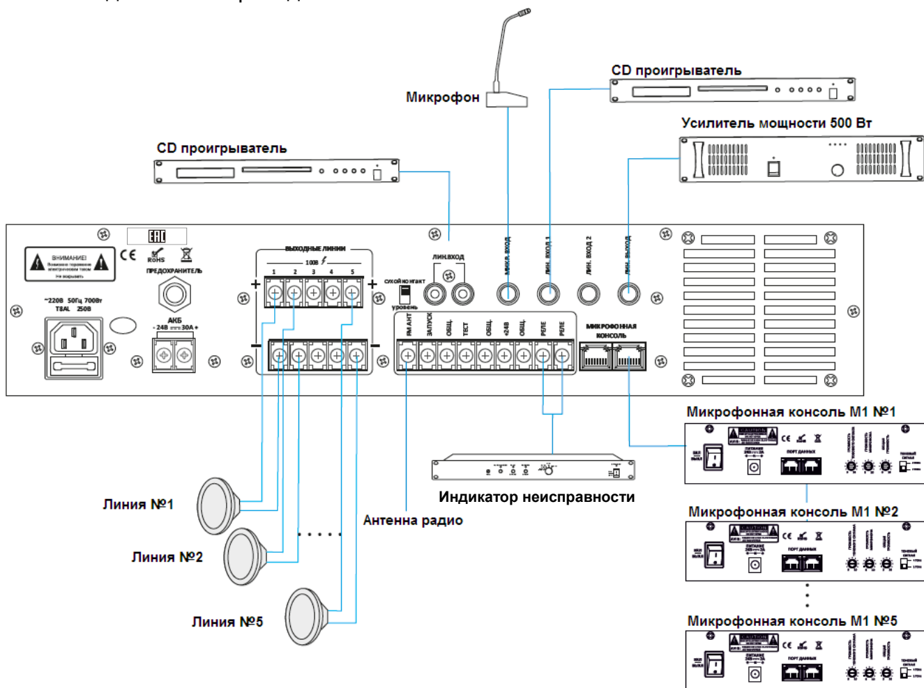
Рис. 2.1 Схема подключения
